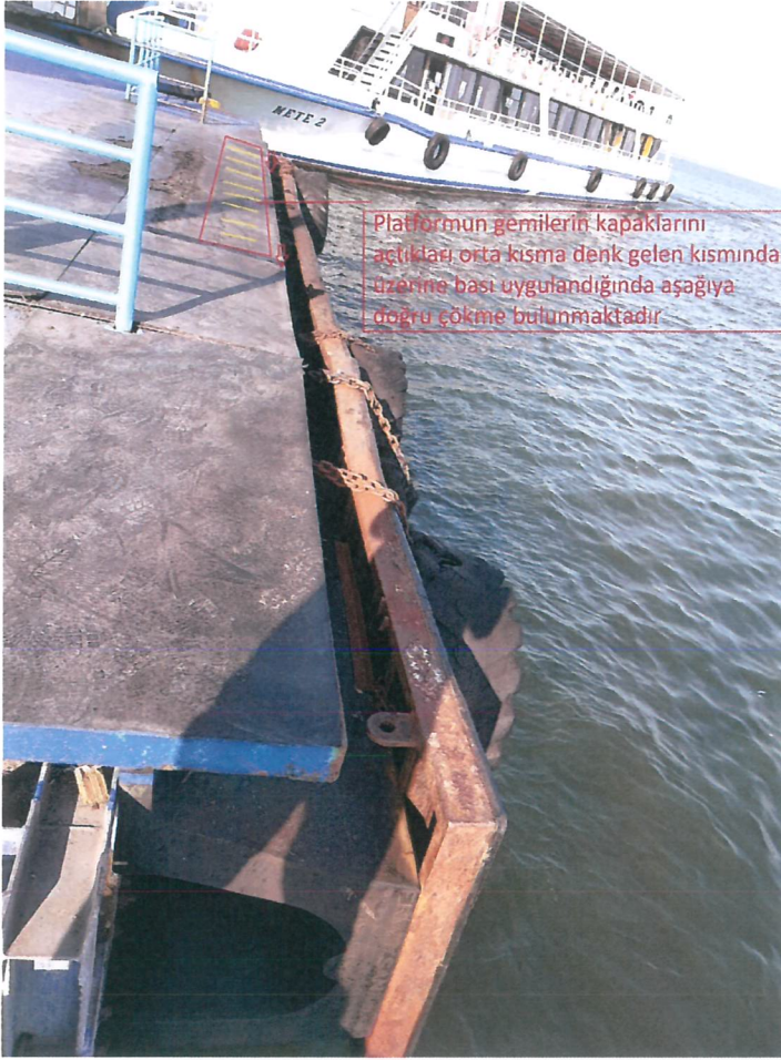
Resim-4. Konak iskelesi Karşıyaka tarafı platform uç kısım zemindeki çökme
