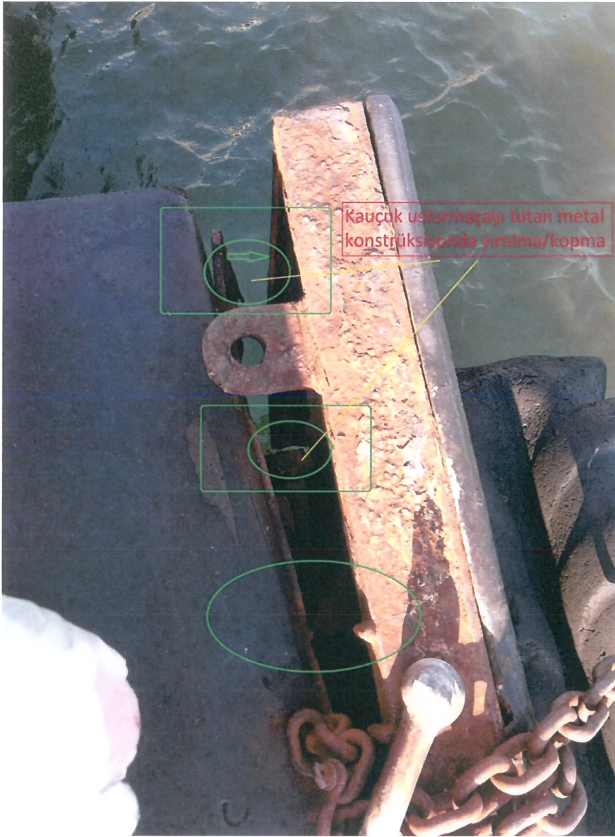
Resim-3. Konak iskelesi Karşıyaka tarafı platform usturmaçalarındaki deformasyon/kırılma ve kopmalar
